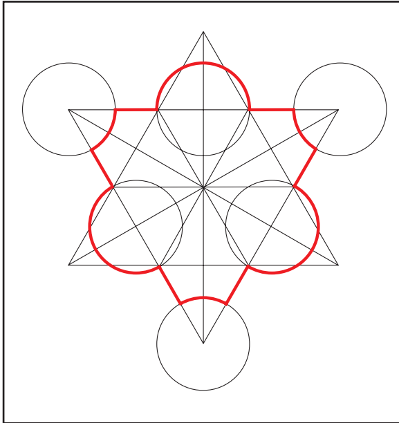
3. kép. A Sant'Ivo alaprajzának szerkesztése
