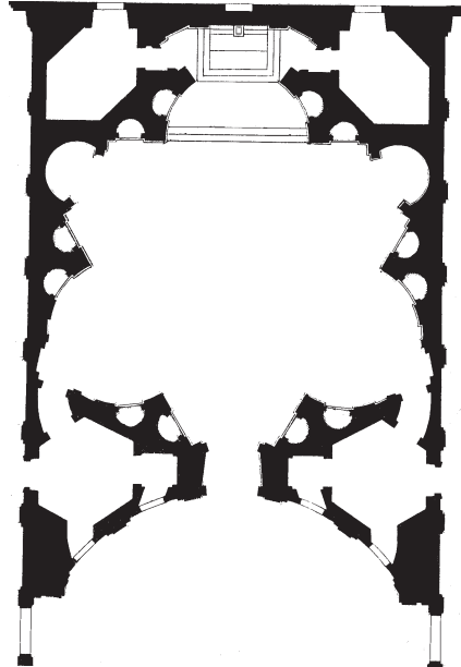
4. kép. A Sant'Ivo alaprajza
