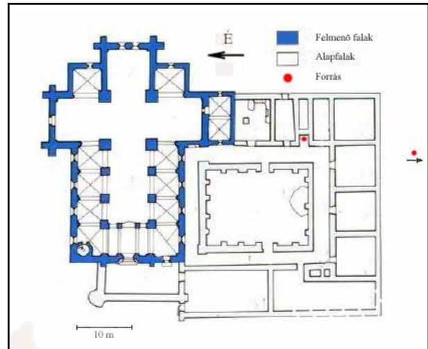
1. kép A templom és a kolostor alaprajza.
